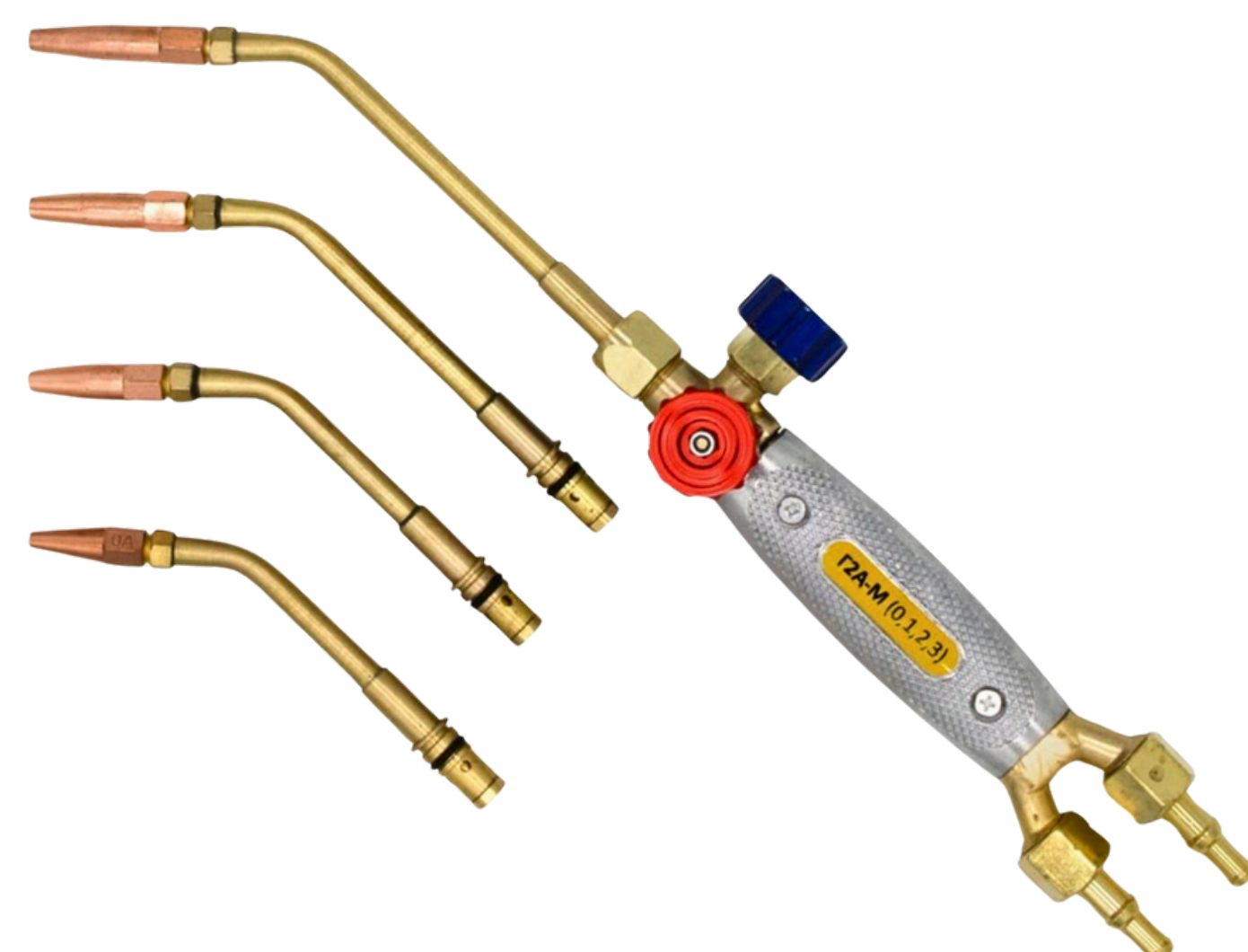
ГОРЕЛКА АЦЕТИЛЕНОВАЯ Г-2А
